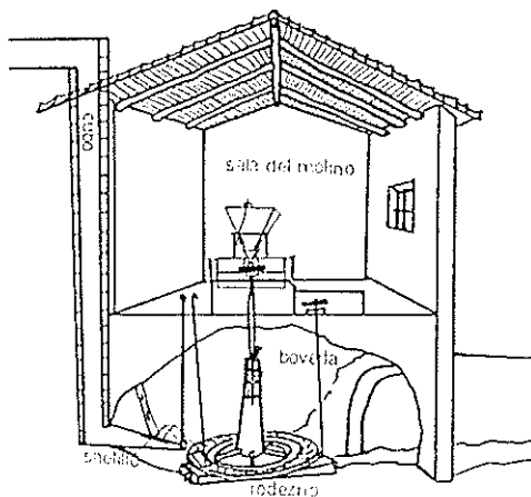
Esquema de molino (de rodete con cubo).
