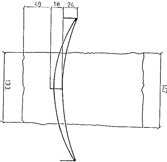
C) PERFIL LATERAL
