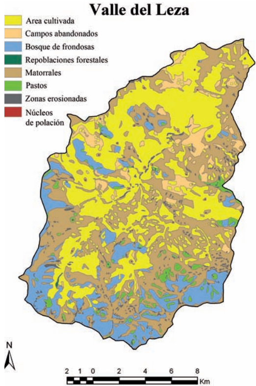
Figura 2: Usos y cubiertas del suelo en el Valle del Leza (1956).
